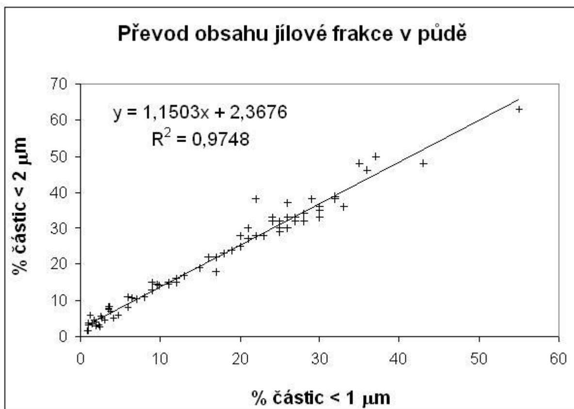
Obr. 2 - Protože v ČR byla stanovována frakce < 1 \mu\text{m} a nikoliv < 2 \mu\text{m} , uvádíme graf umožňující přepočet
