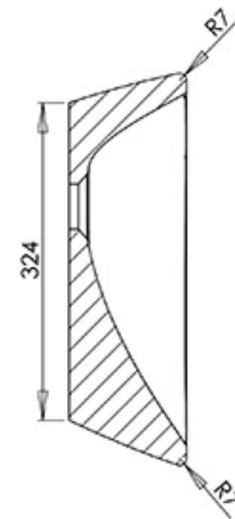
ŘEZ A-A
