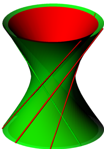
jednodílný hyperboloid
