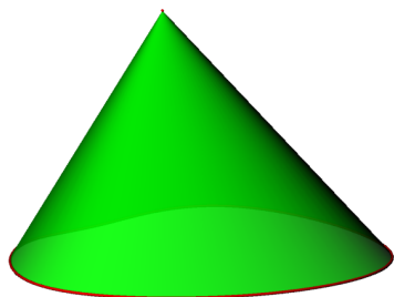
obecný kužel
