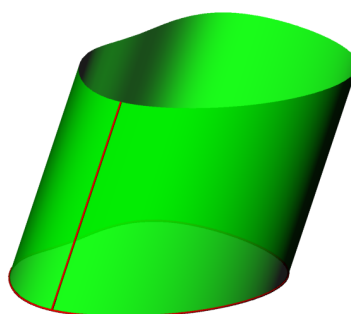
obecný válec
