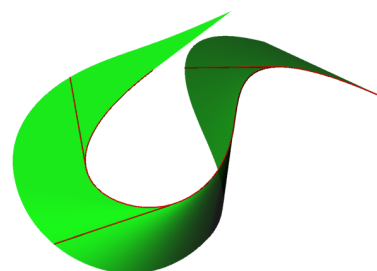
plocha tečen prostorové křivky
