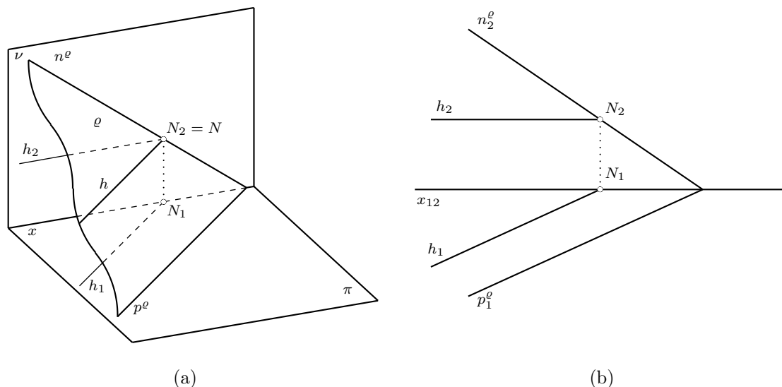
Obrázek 6.14: Horizontální hlavní přímka
