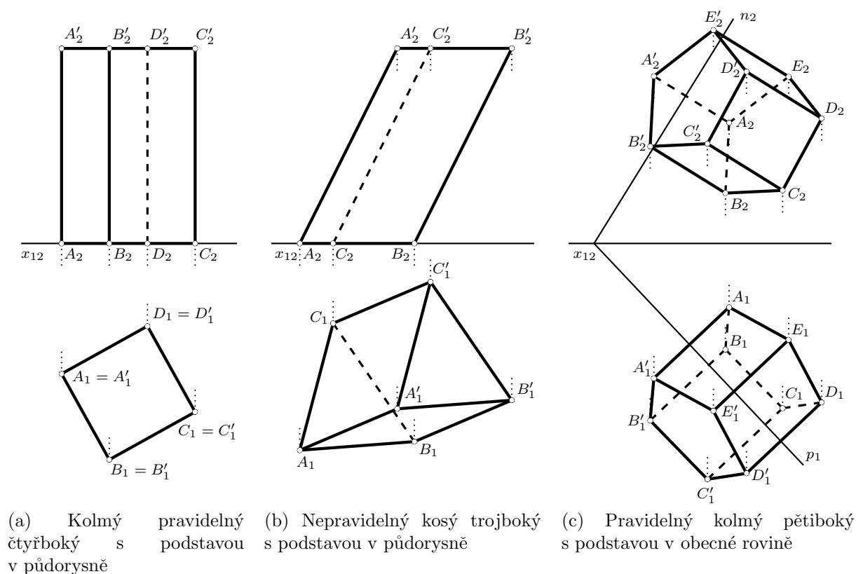
Obrázek 6.28: Hranoly
