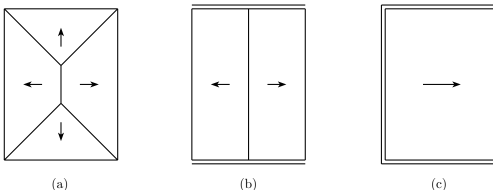
Obrázek 5.16: Od valbové střechy ke střeše pultové
