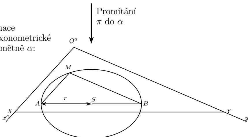
Obrázek 7.9: Vztah mezi kružnicí a elipsou
