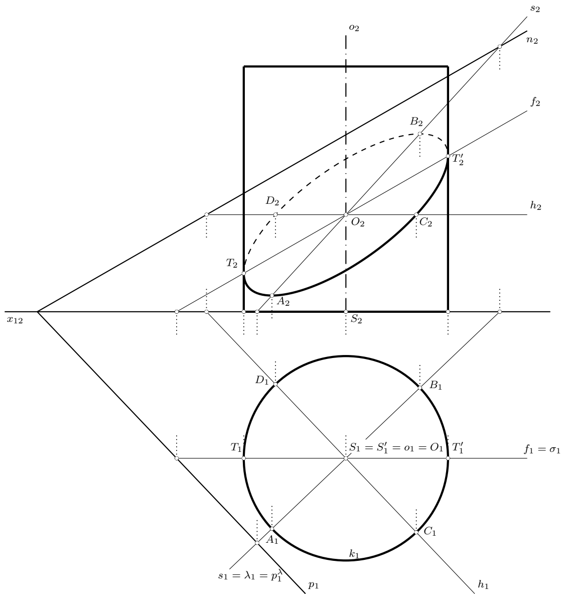
Obrázek 6.39: Řešení příkladu 6.27
