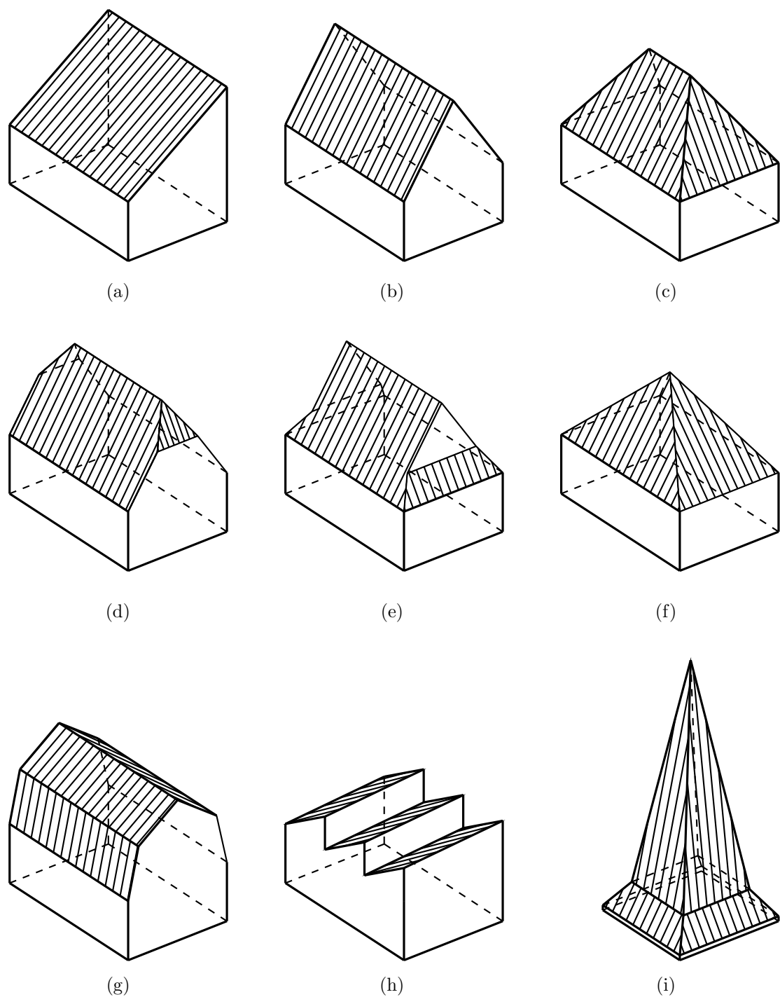
Obrázek 5.3: Rozdělení střech podle tvaru
