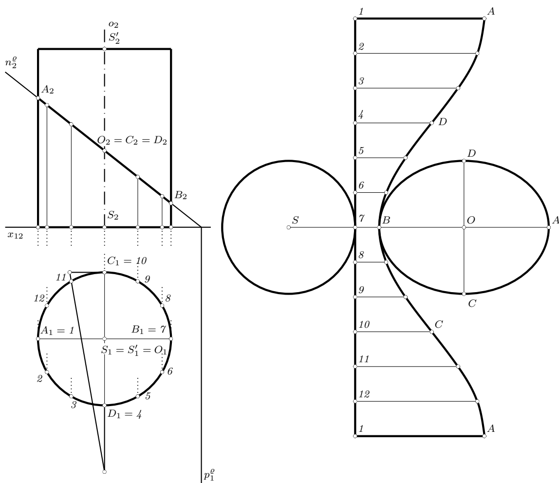
Obrázek 6.38: Řez a síť válce z příkladu 6.26
