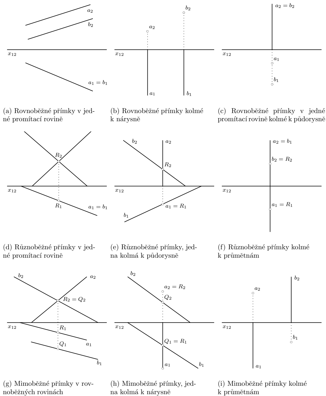
Obrázek 6.8: Vzájemná poloha přímek - speciální polohy
