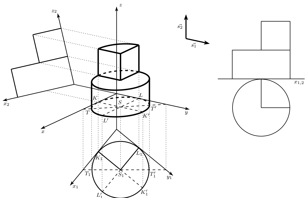
Obrázek 7.44: Zobrazení tělesa zářezovou metodou
