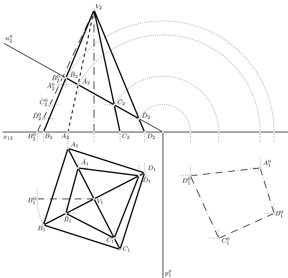
Obrázek 6.34: Řešení příklad 6.22
