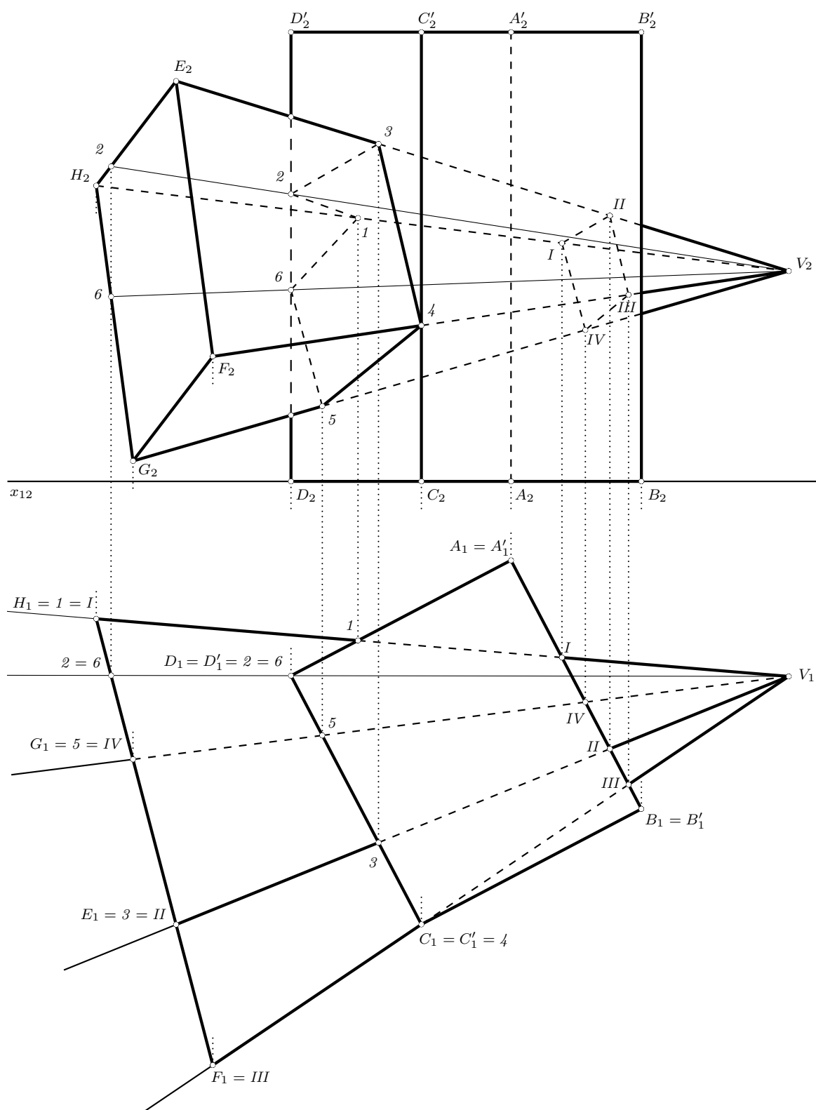
Obrázek 6.56: Průnik jehlanu s hranolem
