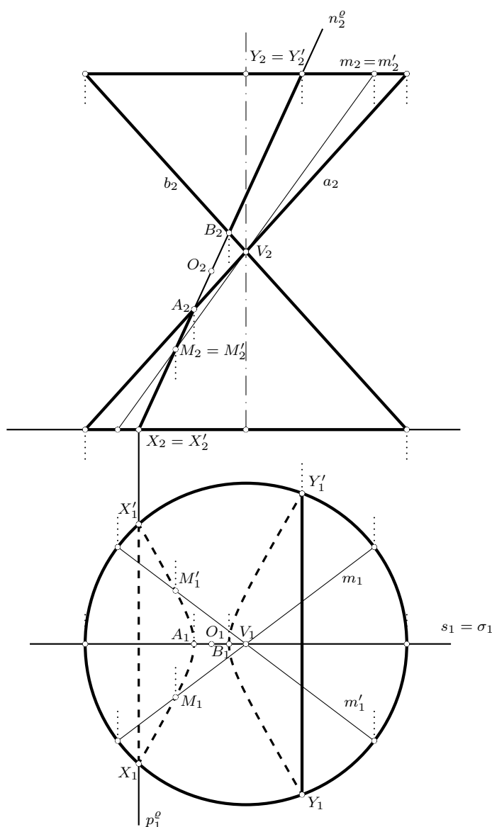
Obrázek 6.45: Řešení příkladu 6.34
