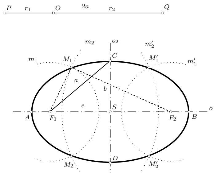
Obrázek 2.1: Elipsa
