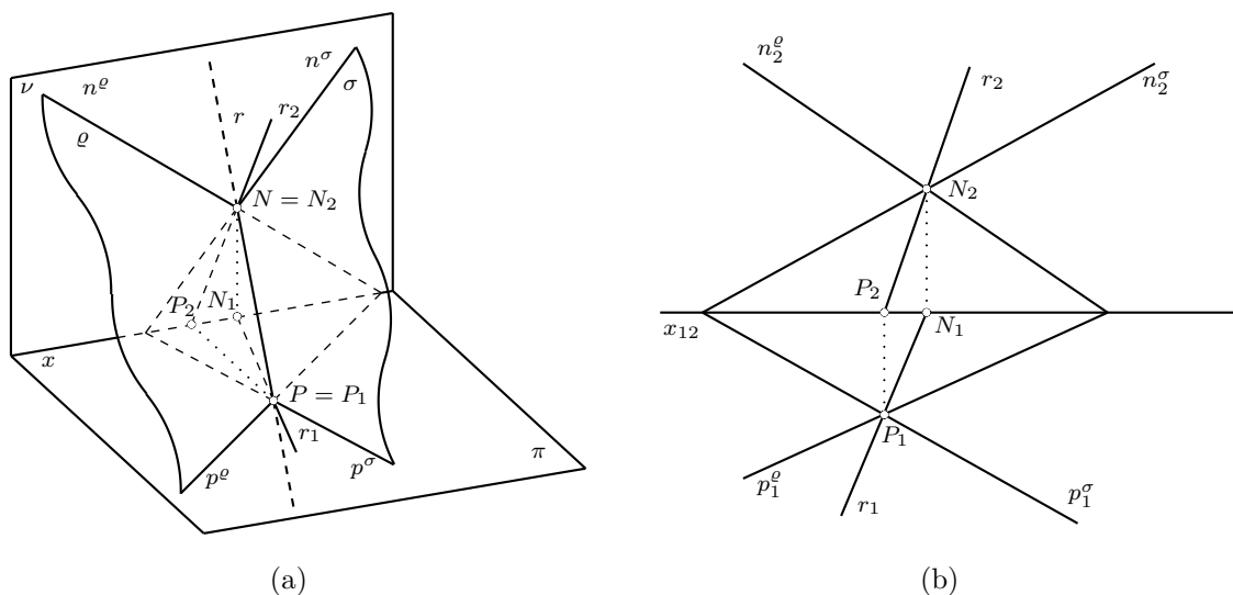
Obrázek 6.18: Průsečnice dvou rovin
