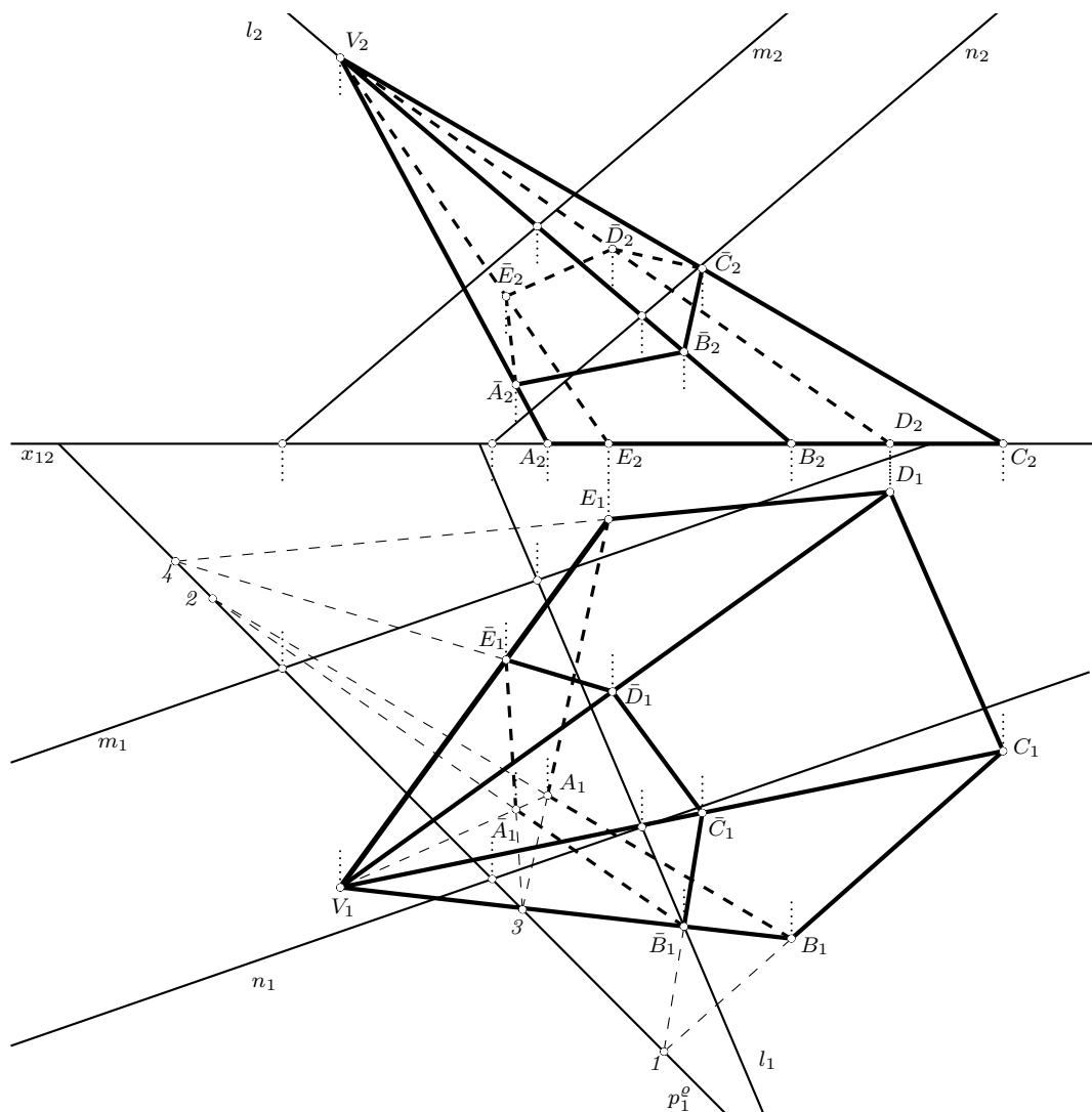
Obrázek 6.36: Řešení příkladu 6.23
