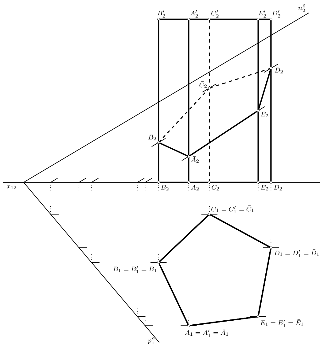
Obrázek 6.29: Řešení příkladu 6.19
