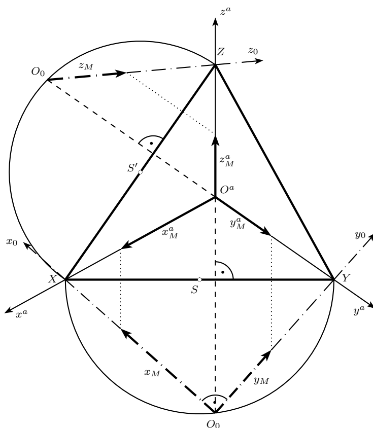
Obrázek 7.6: Otáčení souřadnicových rovin do axonometrické průmětny \alpha
