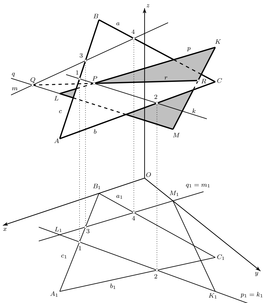
Obrázek 7.25: Vzájemná poloha dvou trojúhelníků
