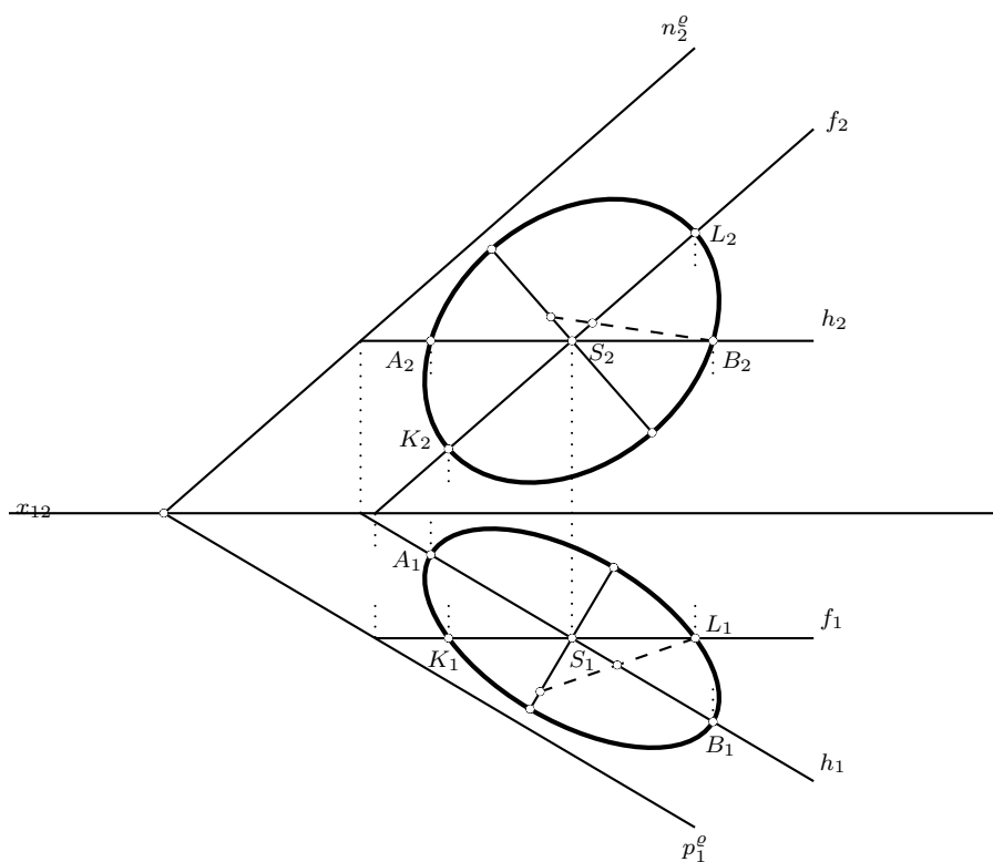
Obrázek 6.27: Zobrazení kružnice
