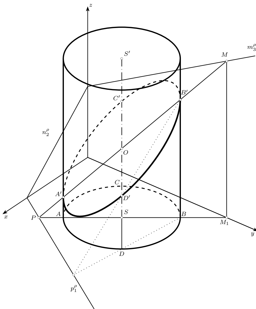
Obrázek 7.31: Řez kolmého válce
