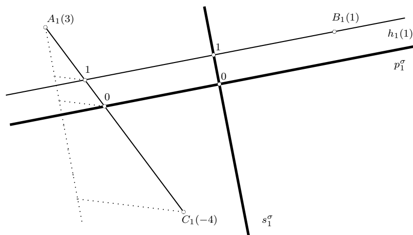
Obrázek 4.16: Řešení příkladu 4.6
