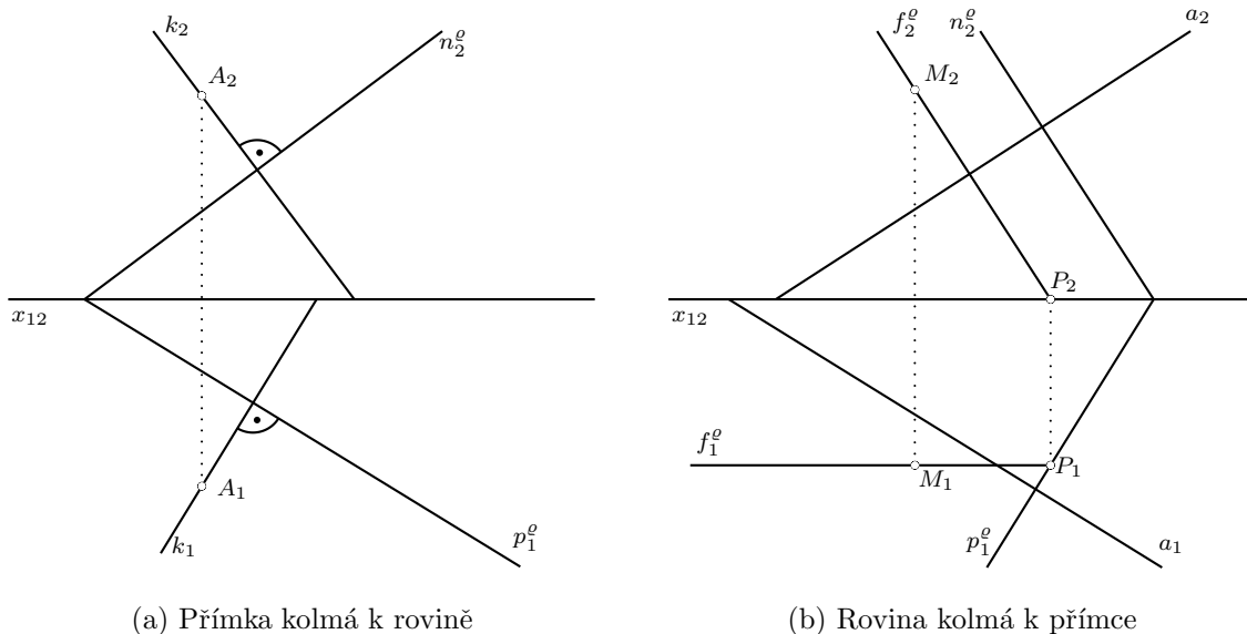
Obrázek 6.23: Kolmost přímek a rovin
