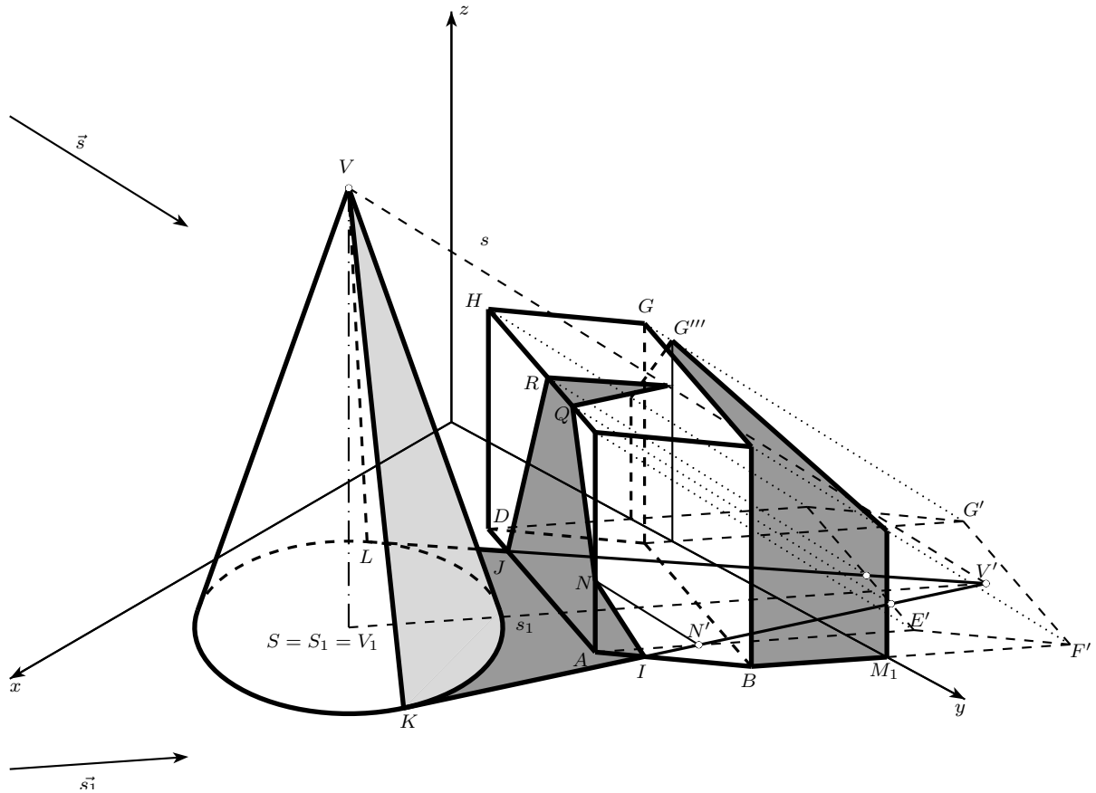
Obrázek 7.42: Vržený stín kužele na hranol
