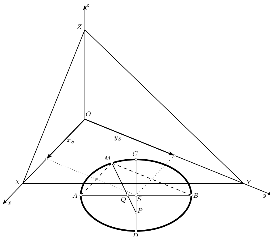
Obrázek 7.8: Zobrazení kružnice v půdorysně
