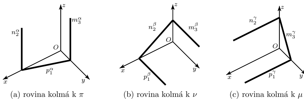
Obrázek 7.16: Roviny kolmé k průmětně
