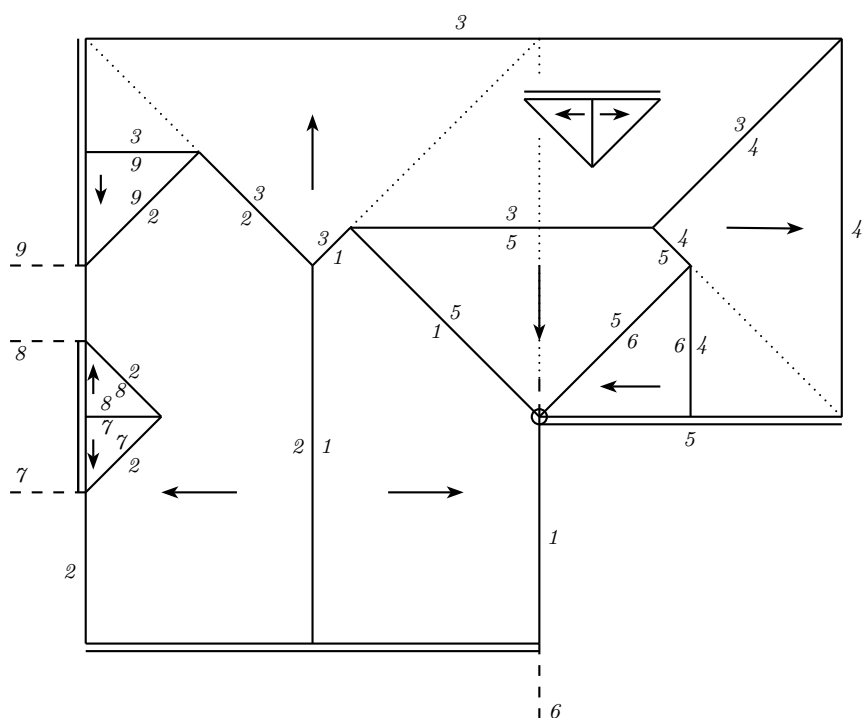
Obrázek 5.18: Použití zakázaných okapů 1
