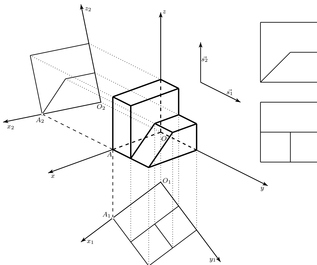
Obrázek 7.43: Zobrazení tělesa zářezovou metodou
