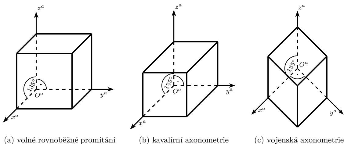
Obrázek 7.4: Speciální typy kosoúhlých axonometrií
