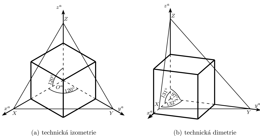
Obrázek 7.5: Speciální typy pravoúhlých axonometrií
