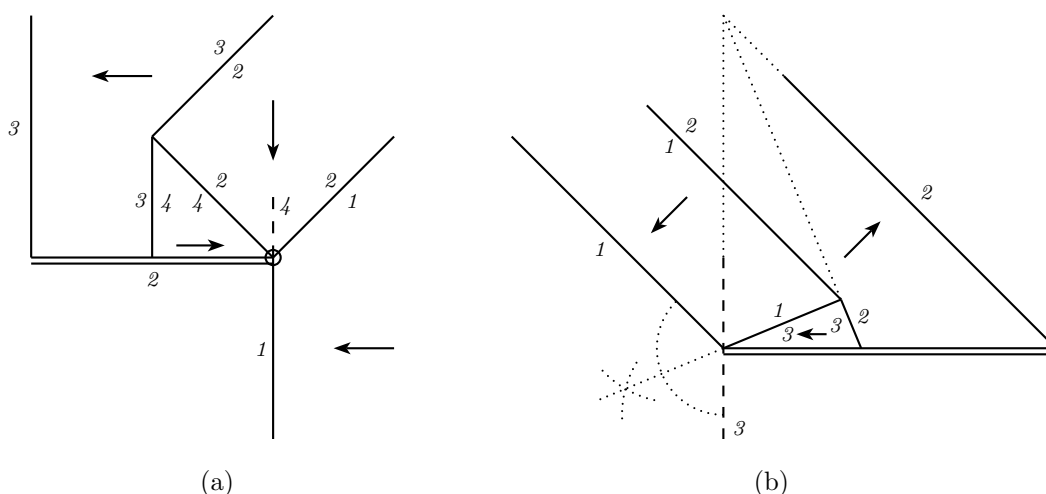
Obrázek 5.17: Další případy zakázaných okapů
