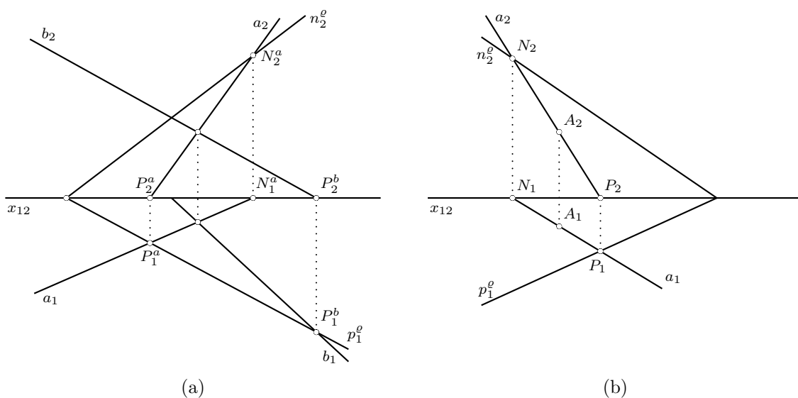
Obrázek 6.13: Řešení příkladů 6.6 a 6.7
