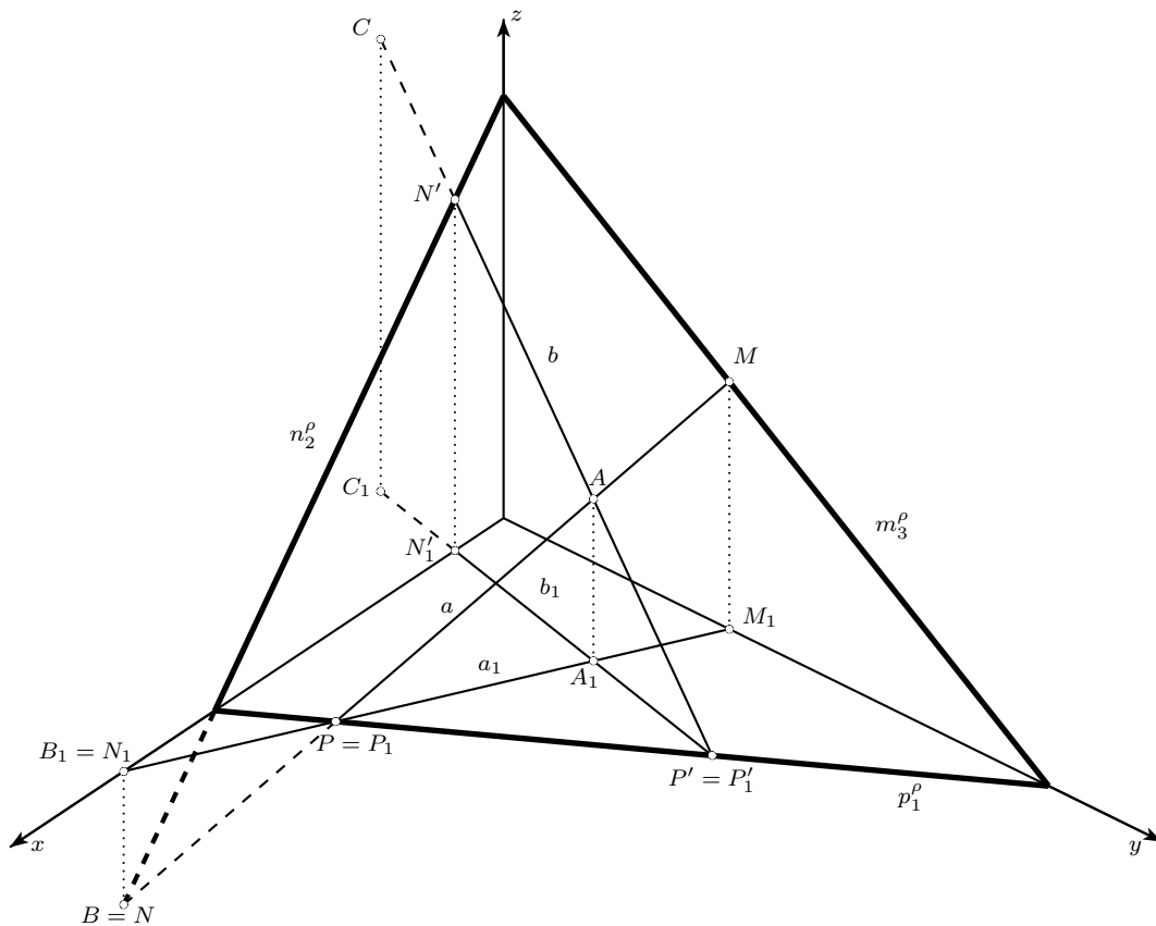
Obrázek 7.12: Stopy roviny
