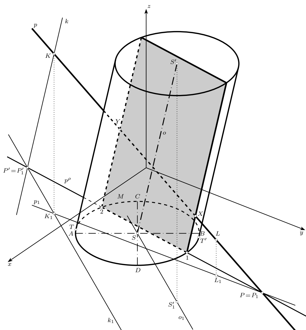
Obrázek 7.34: Průsečíky přímky se šikmým válcem
