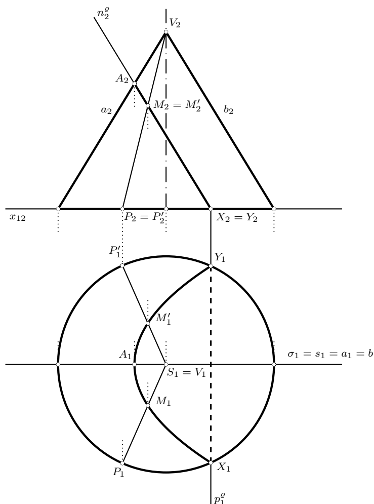
Obrázek 6.44: Řešení příkladu 6.33
