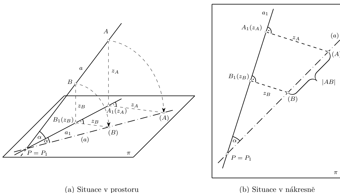
Obrázek 4.7: Sklápění přímky otočením promítací roviny do půdorysny
