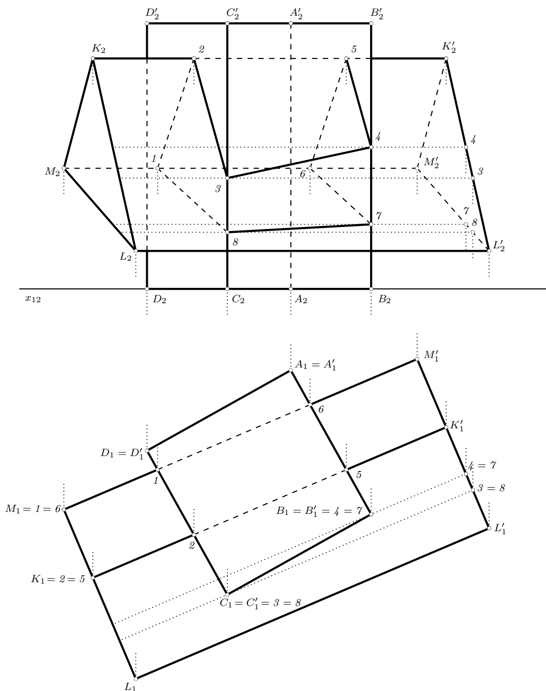
Obrázek 6.55: Průnik dvou hranolů
