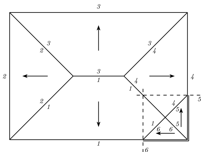
Obrázek 5.21: Zakázané rohy - použití
