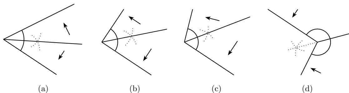
Obrázek 5.5: Průsečnice sousedních střešních rovin
