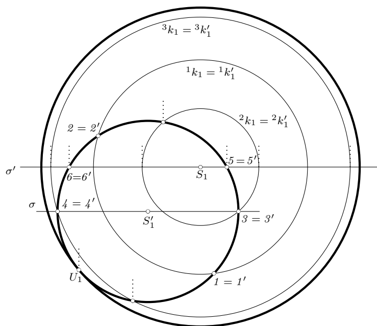
Obrázek 6.57: Průnik válce a koule s dvojným bodem
