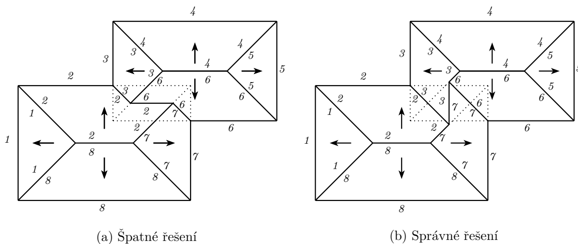
Obrázek 5.9: Střecha s nebezpečím žlabu
