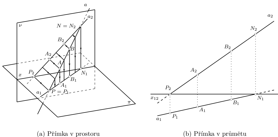
Obrázek 6.4: Zobrazení přímky
