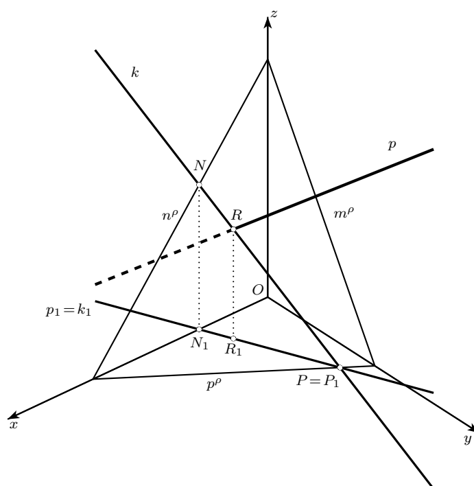
Obrázek 7.21: Průsečík přímky s rovinou
