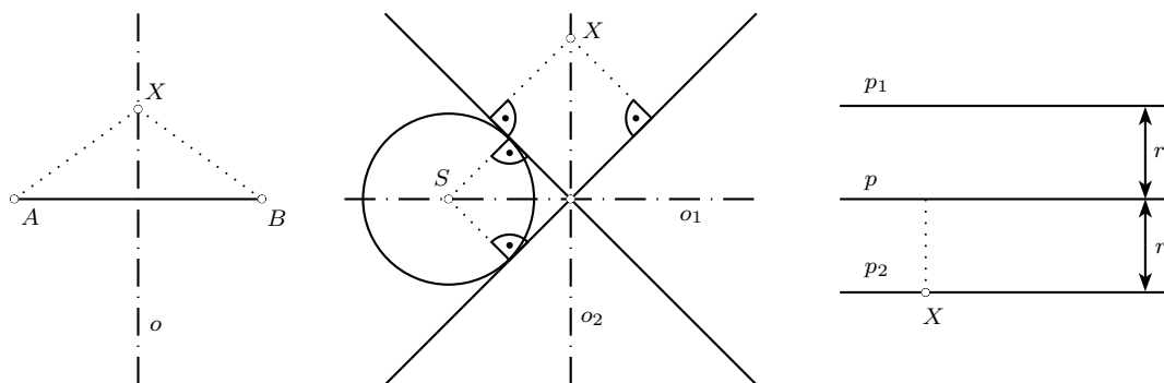
Obrázek 1.2: Základní množiny všech bodů dané vlastností
