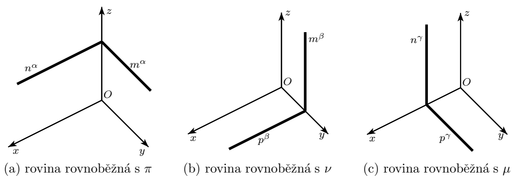
Obrázek 7.15: Roviny rovnoběžné s průmětnou
