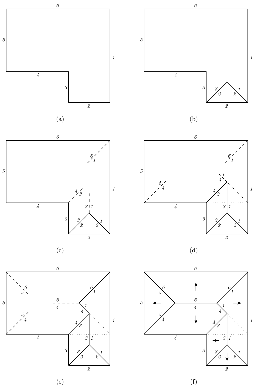
Obrázek 5.8: Číslovací metoda
