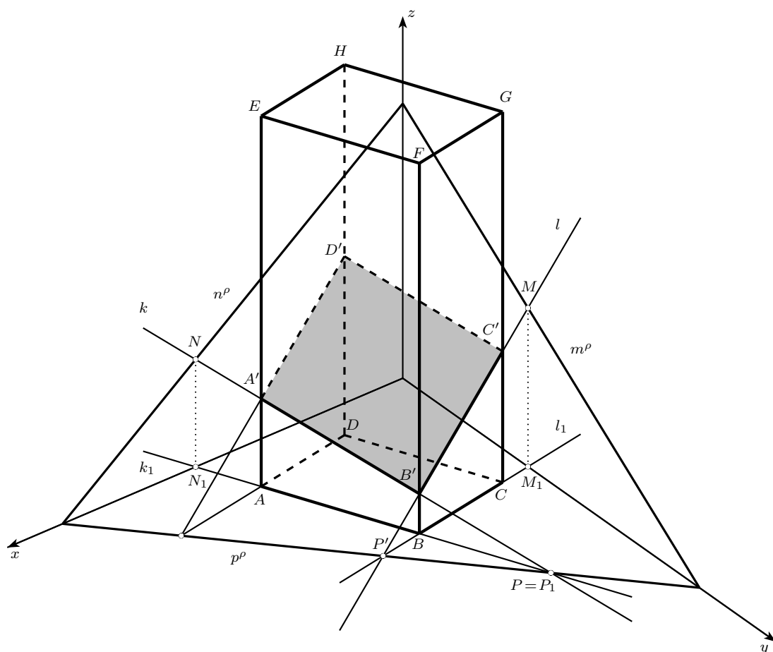
Obrázek 7.27: Řez kolmého hranolu
