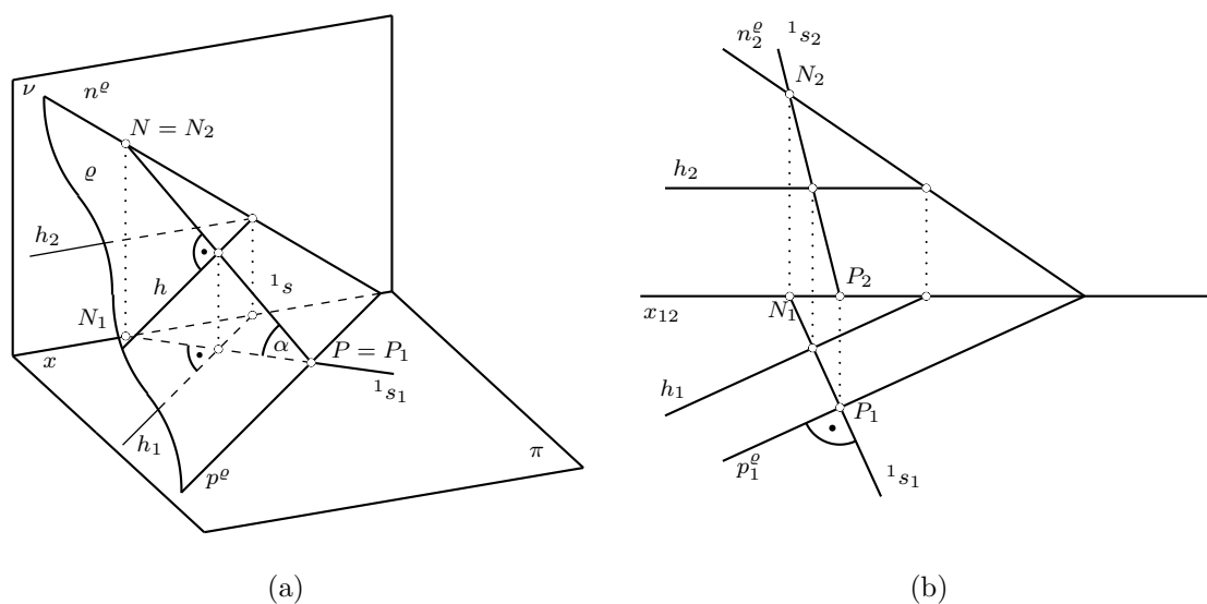
Obrázek 6.16: Spádová přímka první osnovy
