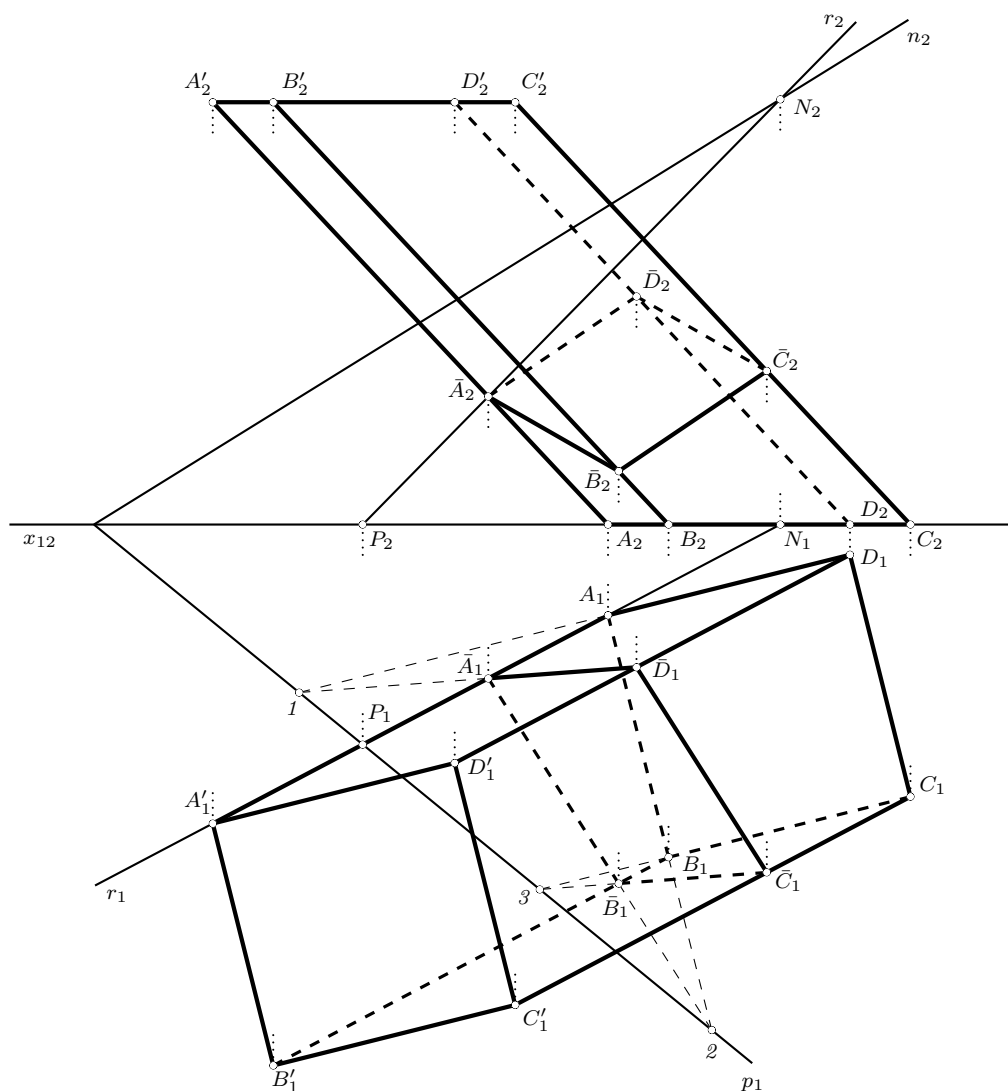
Obrázek 6.30: Řešení příkladu 6.20
