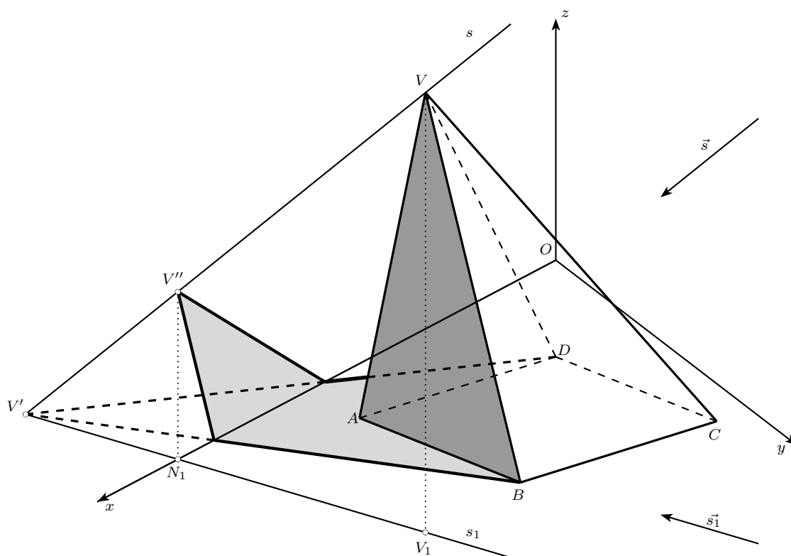
Obrázek 7.37: Rovnoběžné osvětlení šikmého jehlanu
