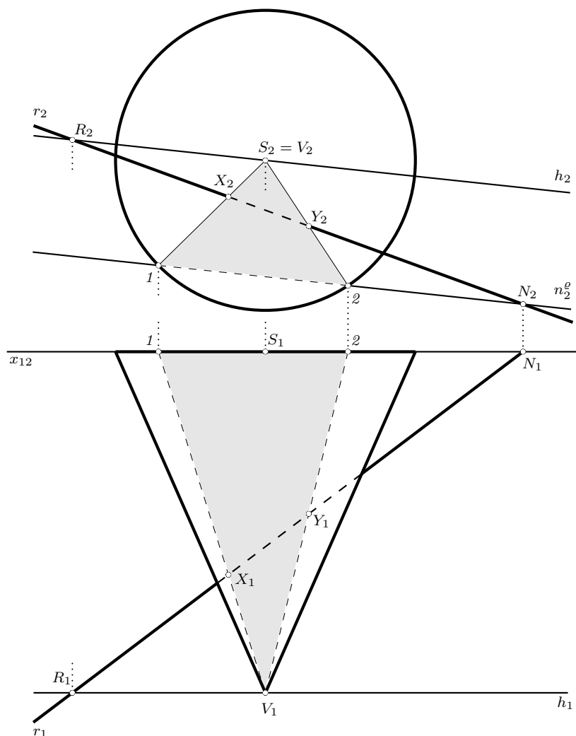
Obrázek 6.52: Řešení příkladu 6.40
