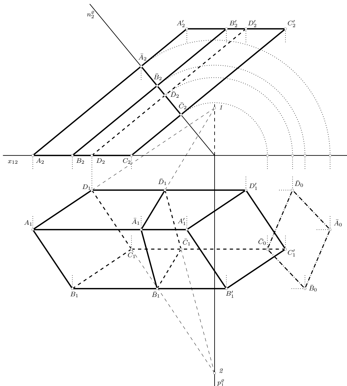
Obrázek 6.31: Řešení příkladu 6.21
