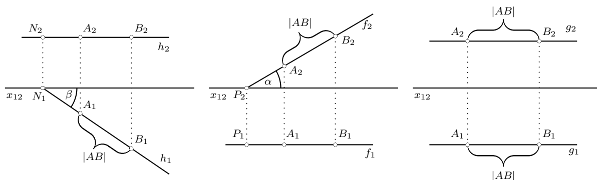
(a) Přímka rovnoběžná s půdorysnou (b) Přímka rovnoběžná s nárysou (c) Přímka rovnoběžná s osou x
