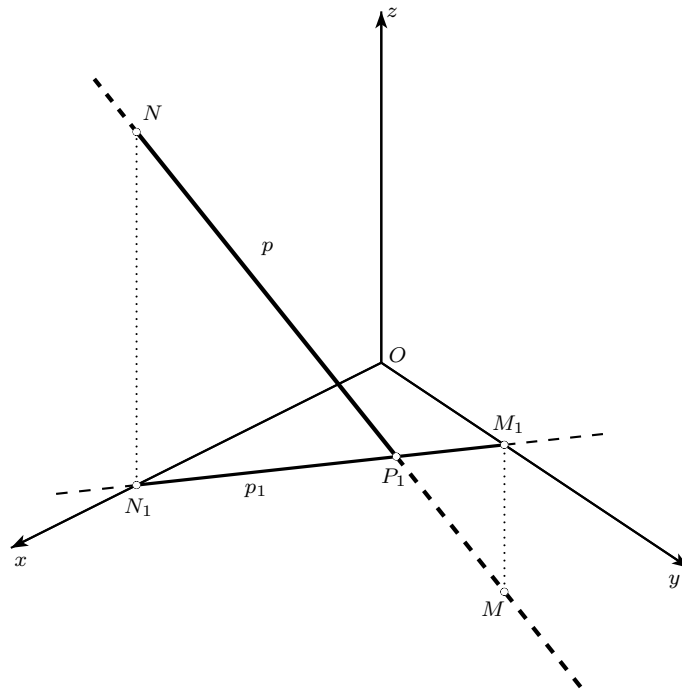
Obrázek 7.10: Stopníky přímky
