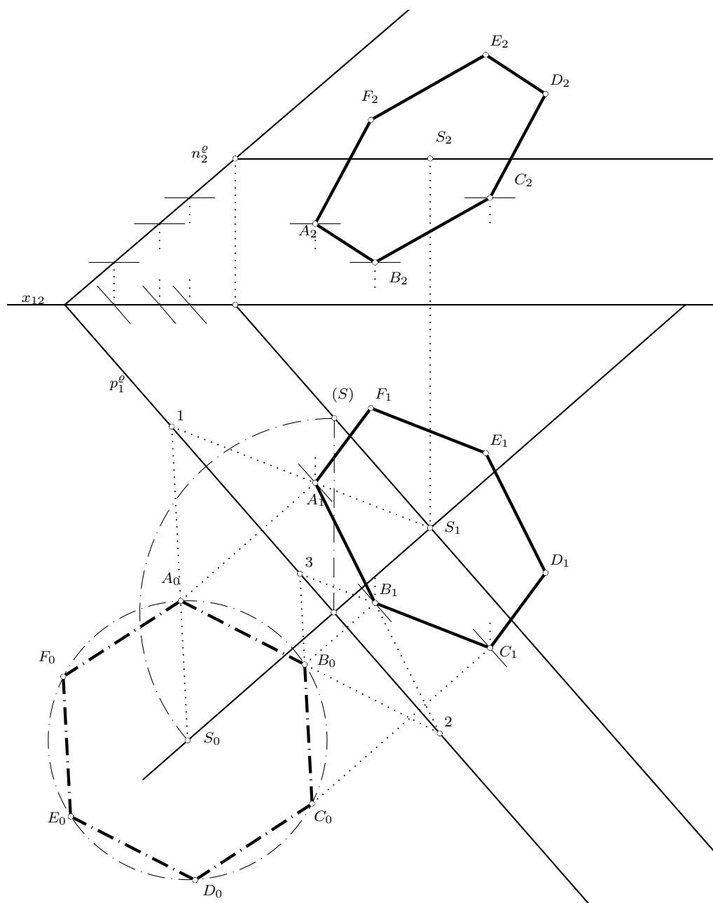
Obrázek 6.26: Konstrukce šestiúhelníku v obecné rovině
