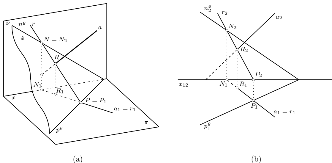
Obrázek 6.21: Průsečík přímky s rovinou
