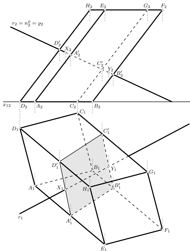
Obrázek 6.48: Řešení příkladu 6.37 pomocí roviny kolmé k nárysně
