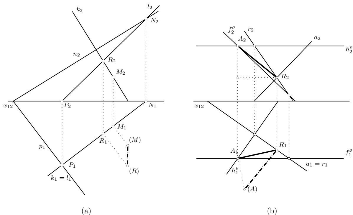
Obrázek 6.24: Určení vzdáleností
