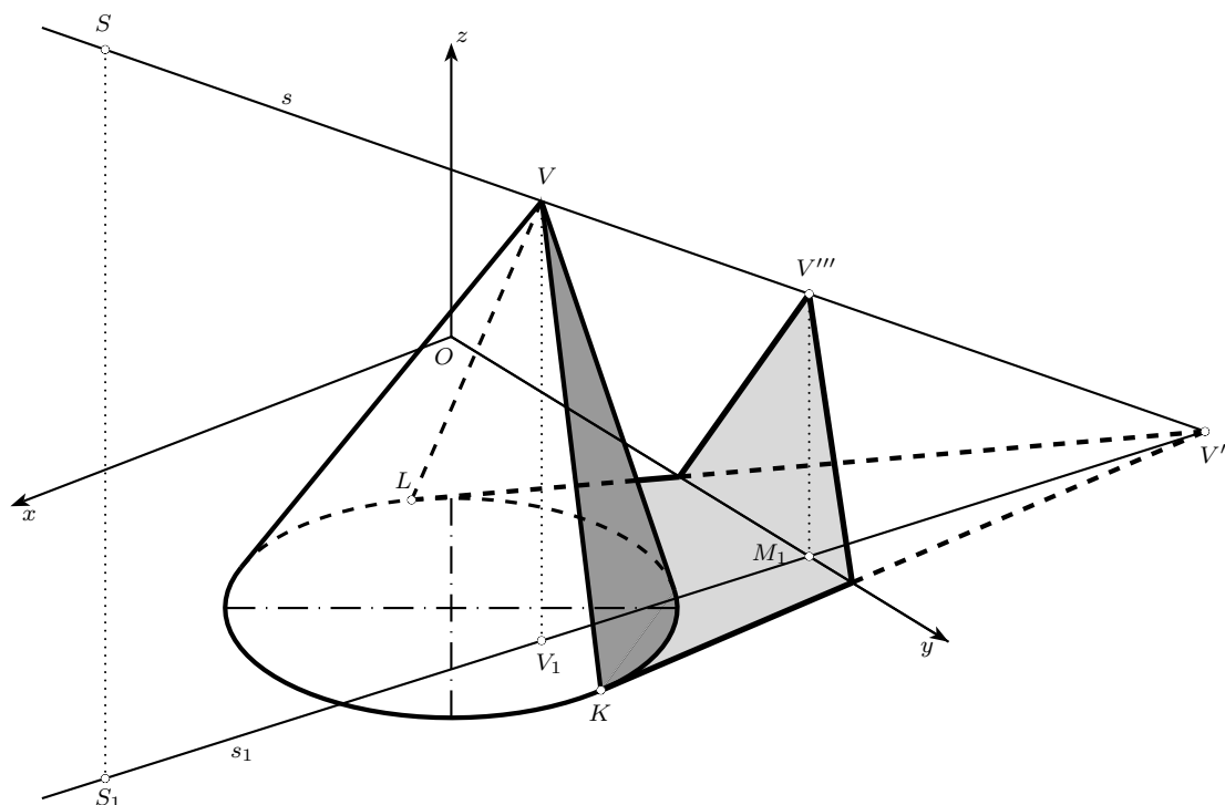
Obrázek 7.38: Středové osvětlení šikmého kužele
