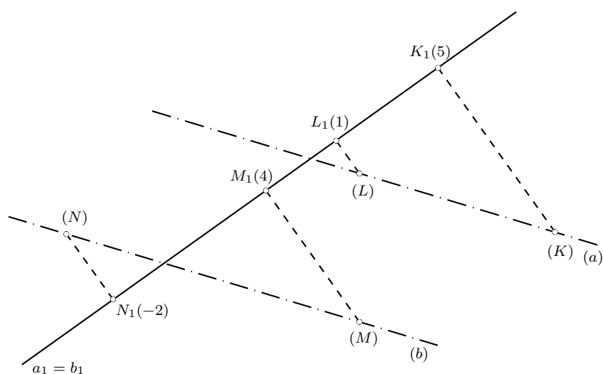
Obrázek 4.14: Řešení příklad 4.5
