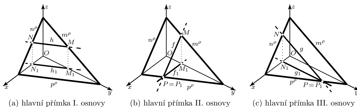
Obrázek 7.13: Hlavní přímky roviny
