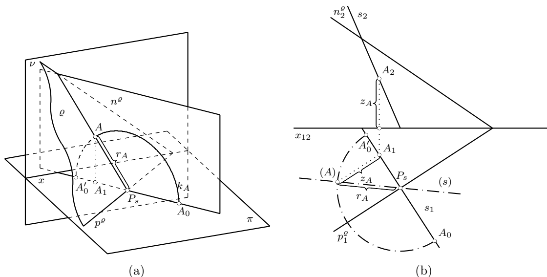
Obrázek 6.25: Otáčení roviny
