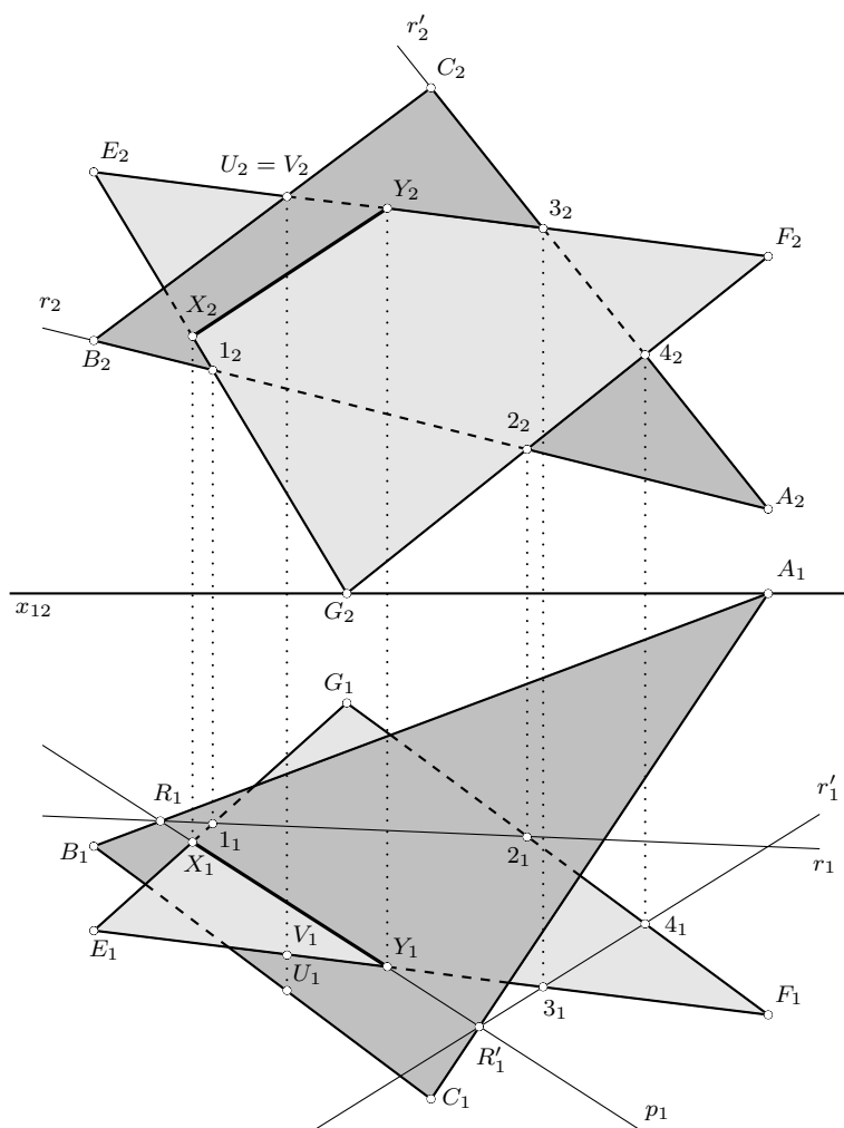
Obrázek 6.22: Průnik dvou trojúhelníků
