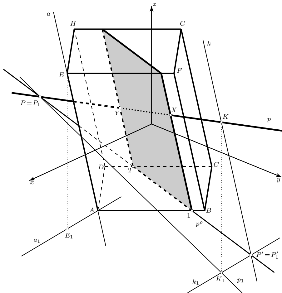
Obrázek 7.33: Průsečíky přímky se šikmým hranolem
