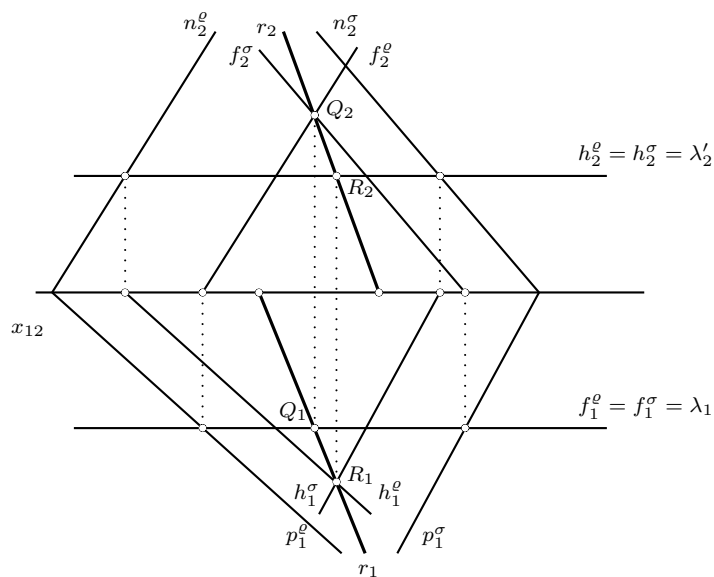
Obrázek 6.19: Řešení příkladu 6.9
