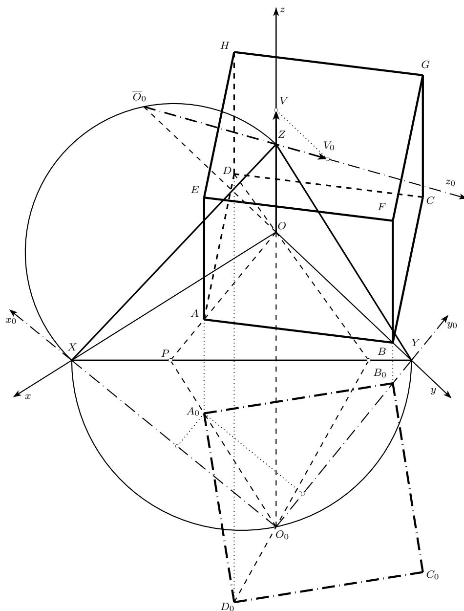
Obrázek 7.7: Zobrazení krychle v kolmé axonometrii
