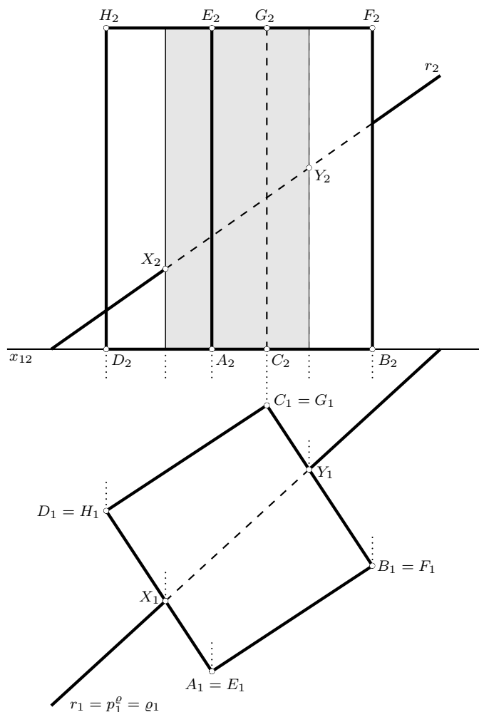
Obrázek 6.47: Řešení příkladu 6.36
