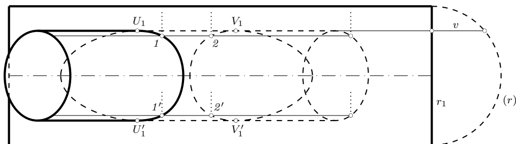
Obrázek 6.60: Průnik dvou válců
