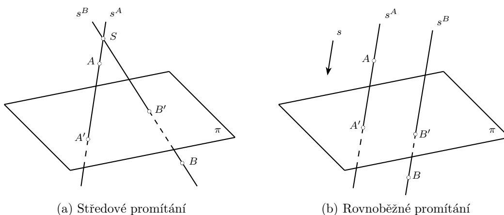
Obrázek 3.1: Princip promítání
