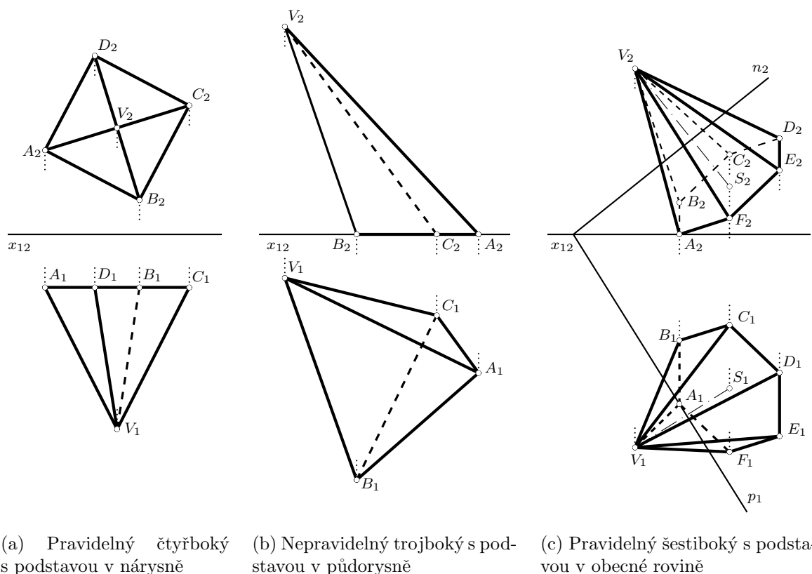
Obrázek 6.33: Jehlany
