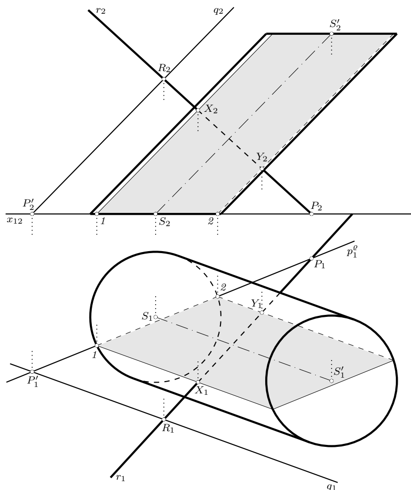
Obrázek 6.50: Řešení příkladu 6.38 pomocí roviny rovnoběžné s osou
