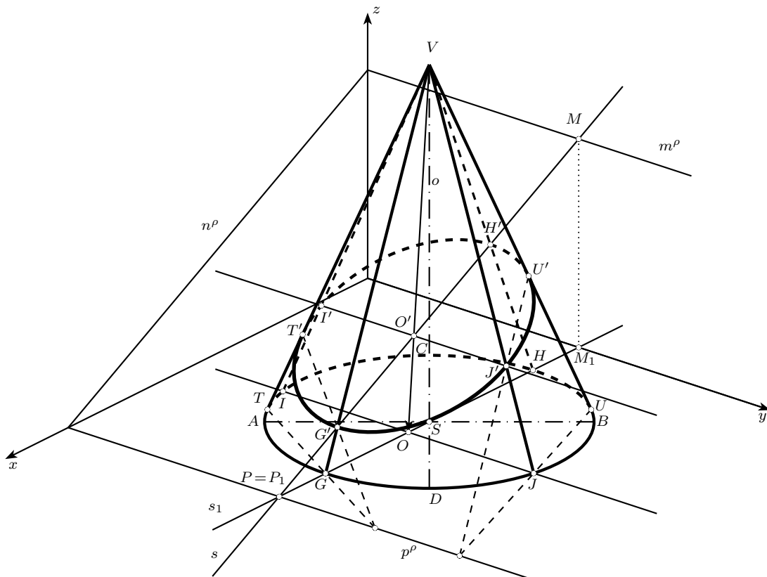
Obrázek 7.32: Eliptický řez rotačního kužele
