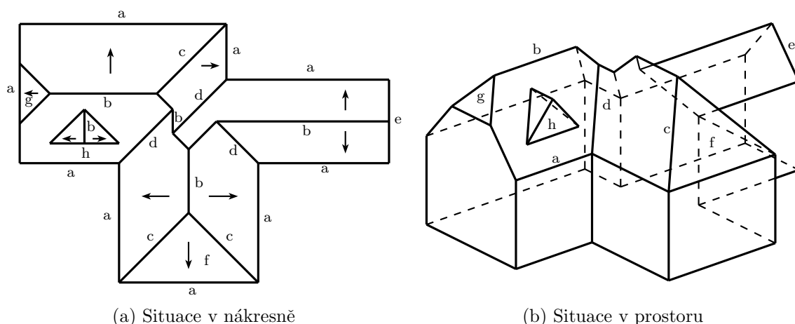
Obrázek 5.1: Názvy hlavních částí sklonité střechy: a - okap, b - hřeben, c - nároží, d - úžlabí, e - štít, f - valba, g - polovalba, h - vikýř, i - roh střechy, j - kout střechy
