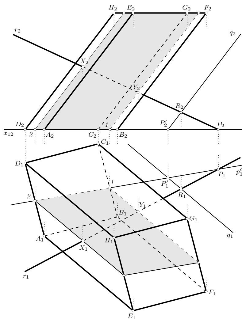
Obrázek 6.49: Řešení příkladu 6.37 pomocí roviny rovnoběžné s hranami
