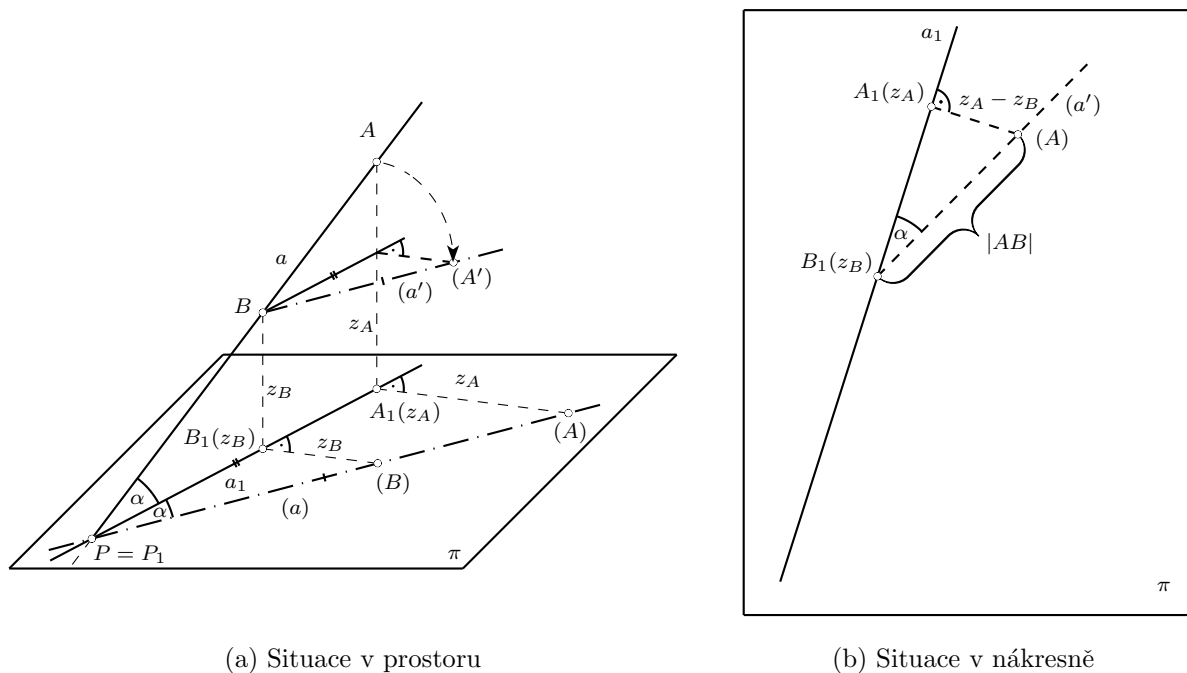
Obrázek 4.8: Sklápění přímky do roviny rovnoběžné s průmětnou
