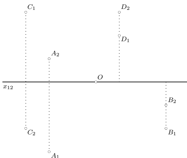
Obrázek 6.3: Řešení příklad 6.1
