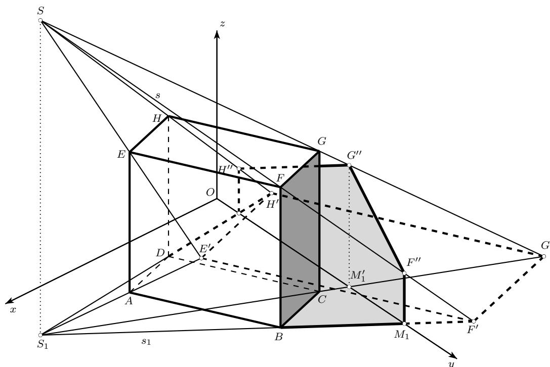
Obrázek 7.40: Středové osvětlení kolmého hranolu
