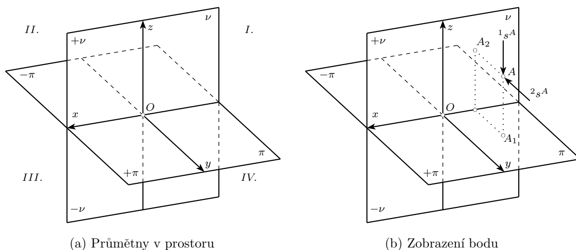
Obrázek 6.1: Mongeovo promítání v prostoru
