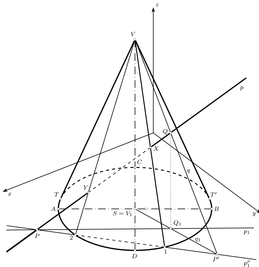
Obrázek 7.36: Průsečíky přímky s kuželem
