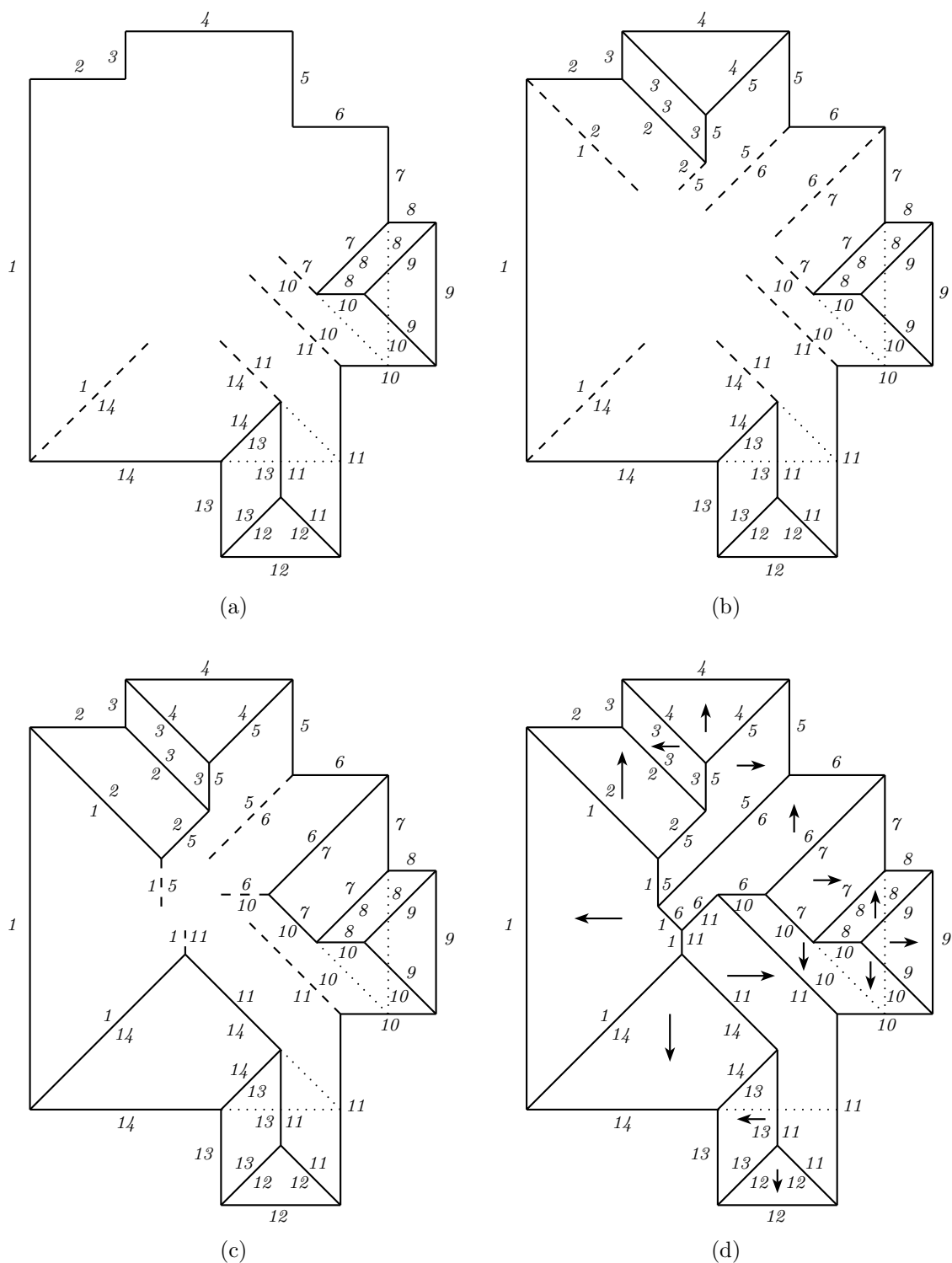
Obrázek 5.11: Postupné řešení střechy nad daným půdorysem
