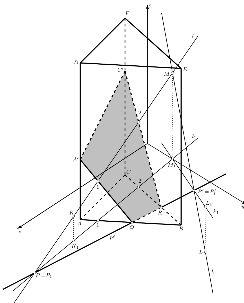
Obrázek 7.28: Řez kolmého hranolu
