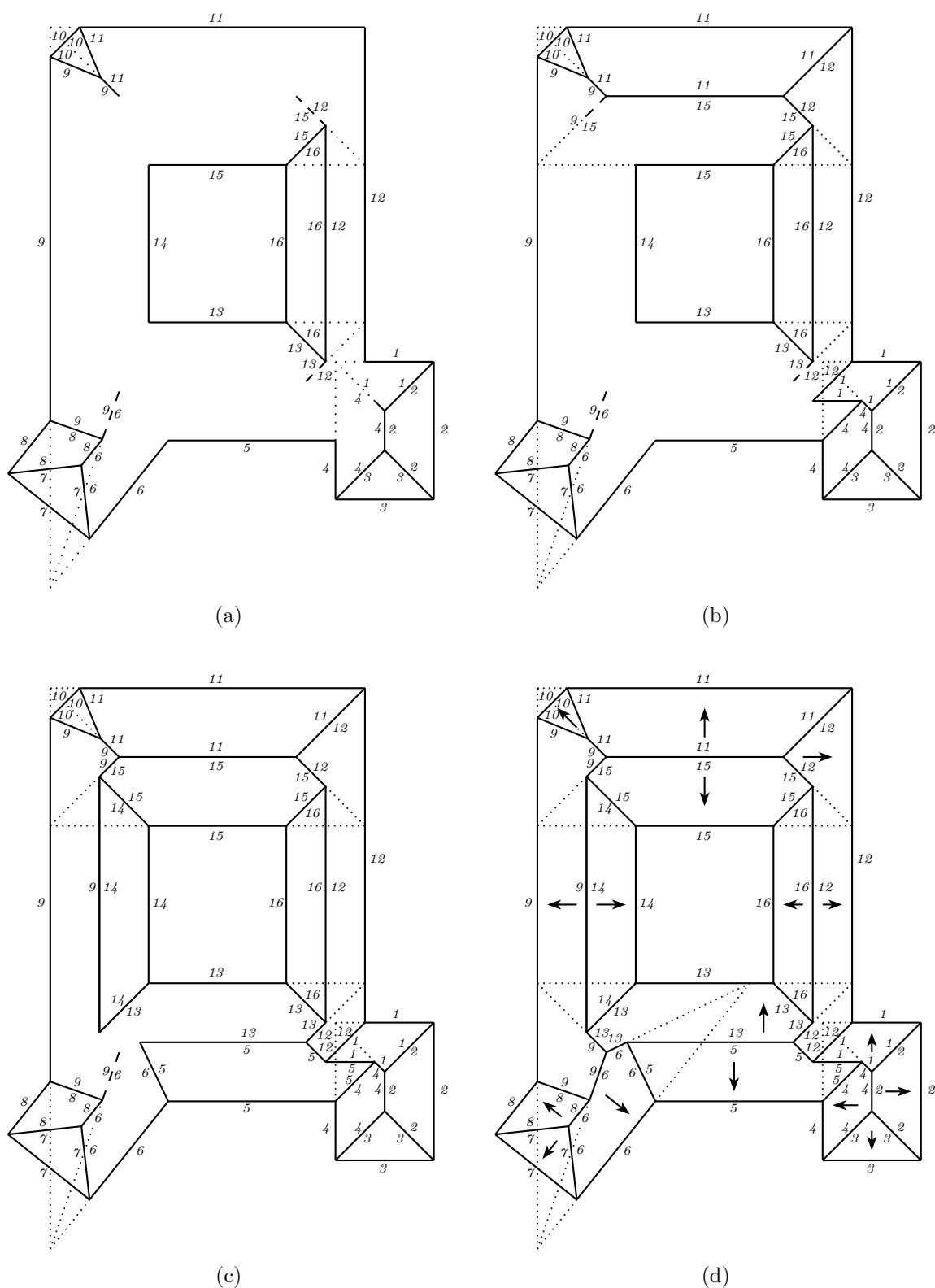
Obrázek 5.12: Postupné řešení střechy s dvorem
