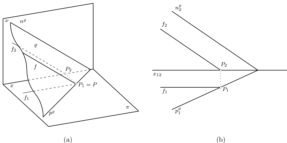
Obrázek 6.15: Frontální hlavní přímka
