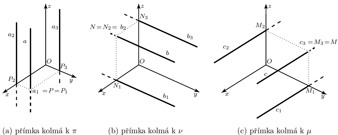
Obrázek 7.14: Přímky kolmé k průmětně
