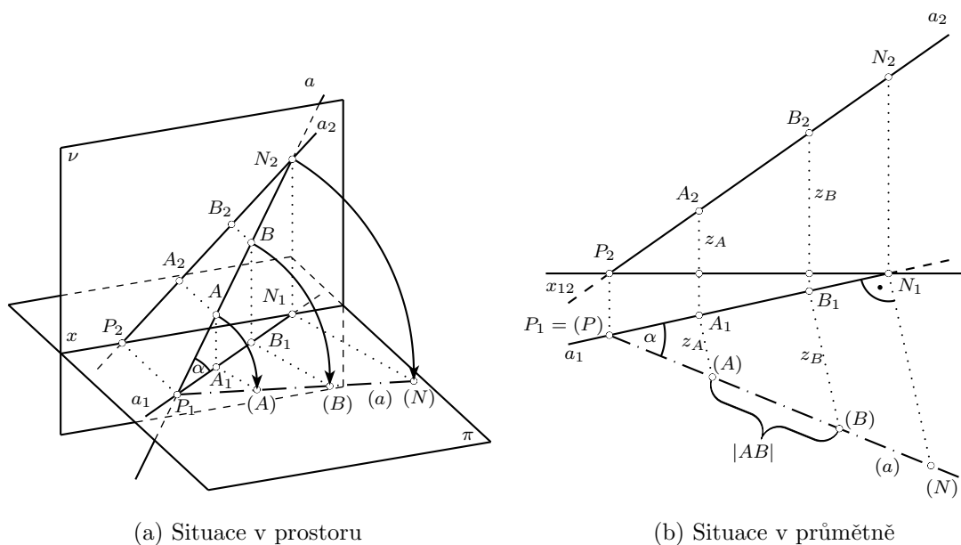
Obrázek 6.5: Sklopení přímky
