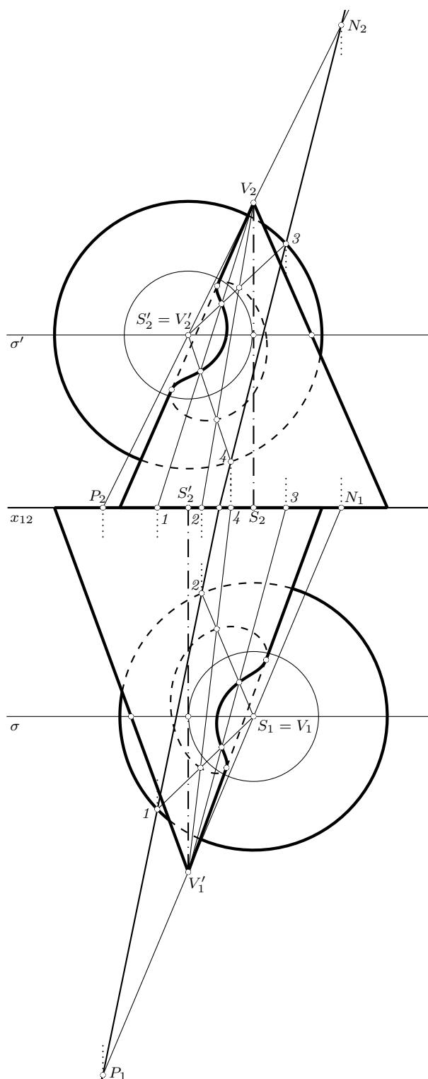
Obrázek 6.61: Průnik kuželů
