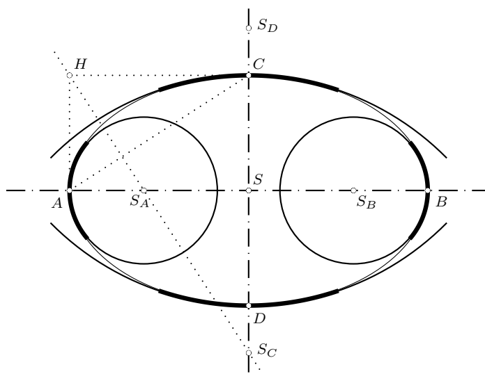
Obrázek 2.2: Hyperoskulační kružnice elipsy
