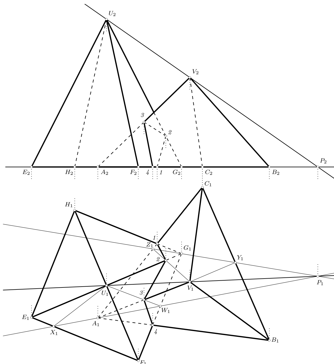
Obrázek 6.54: Průnik dvou jehlanů
