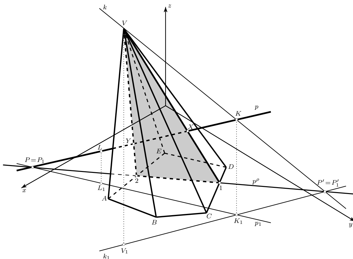
Obrázek 7.35: Průsečíky přímky se šikmým jehlanem
