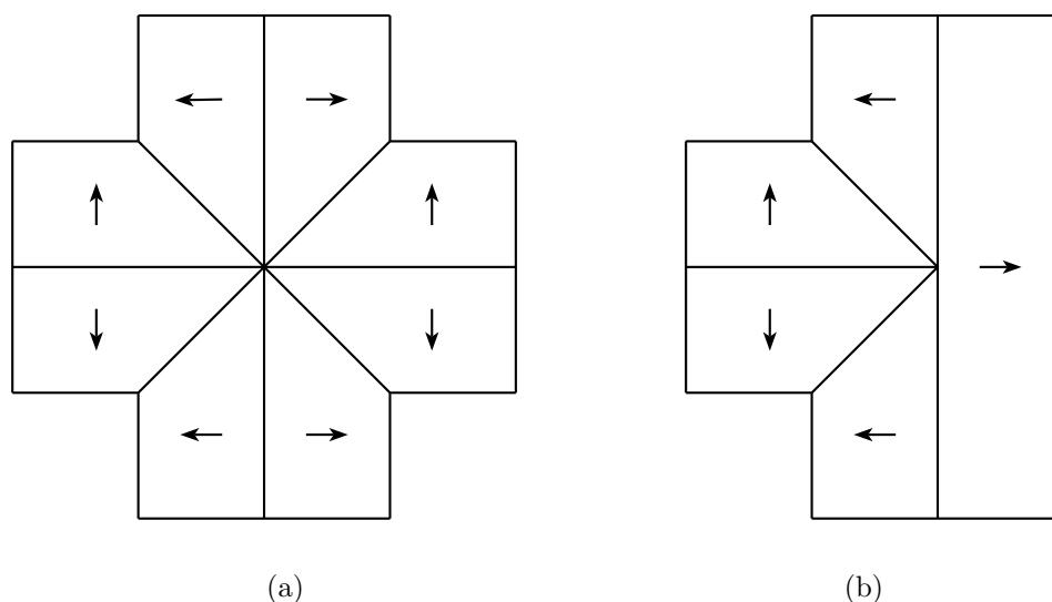
Obrázek 5.4: Střecha křížová, Střecha polokřížová
